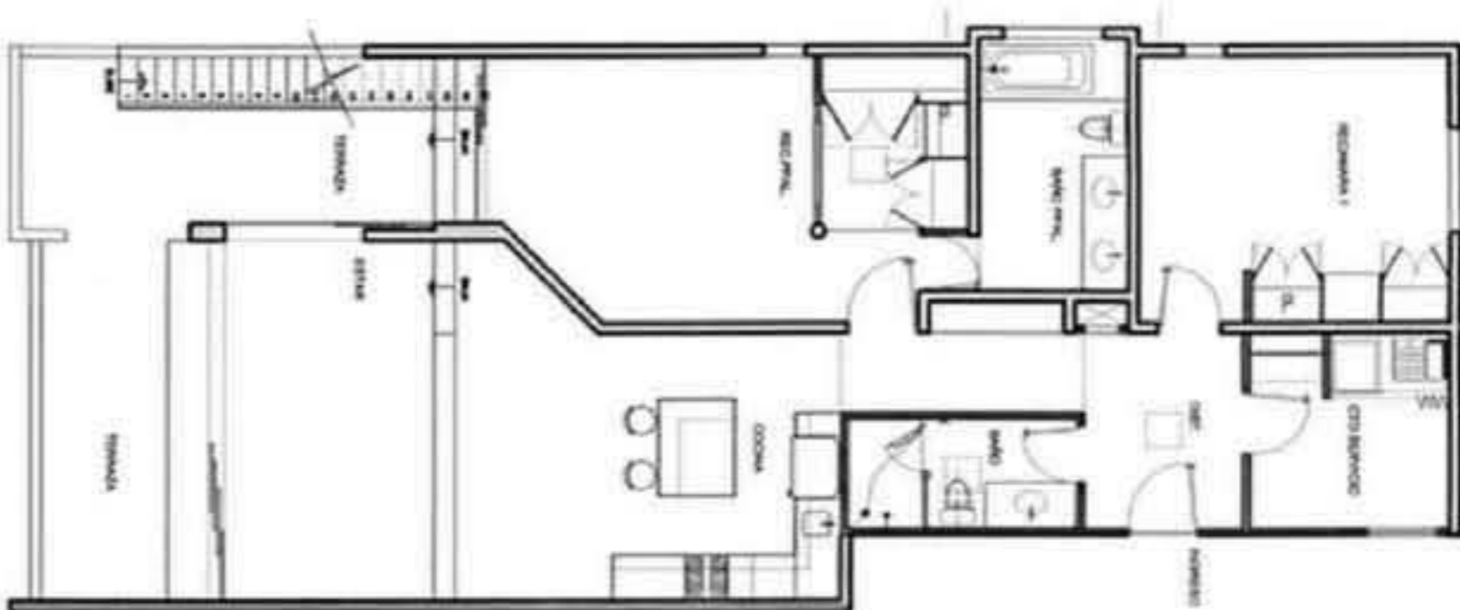
2do nivel. Tipo C 158.34 m 2
